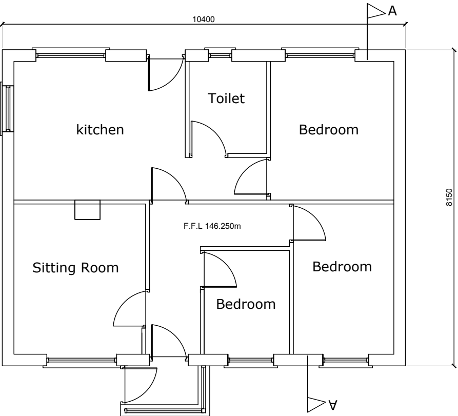
PLAN SCALE; 1:100
